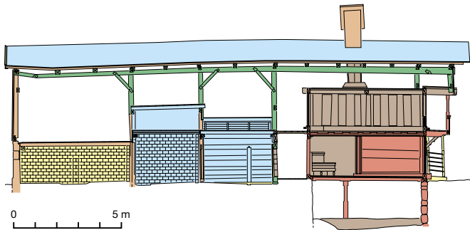
Längsschnitt durch das Tätschdachhaus an der Junkerngasse 17 vor dem Abbau 2014.
