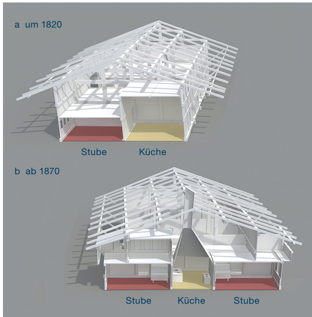
Schwarzenburg, Junkerngasse 17, Grafische Darstellung der Hauskonstruktion und der vermuteten Raumgliederung im Wohnteil. a Zeitstufe I: nach 1574 bis um 1820; b Zeitstufe III: vor 1870 bis 1891.
